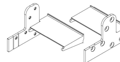
Threshold Wedge 221013.0000.L - 221013.0000.R
